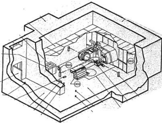
Linear Accelerator
